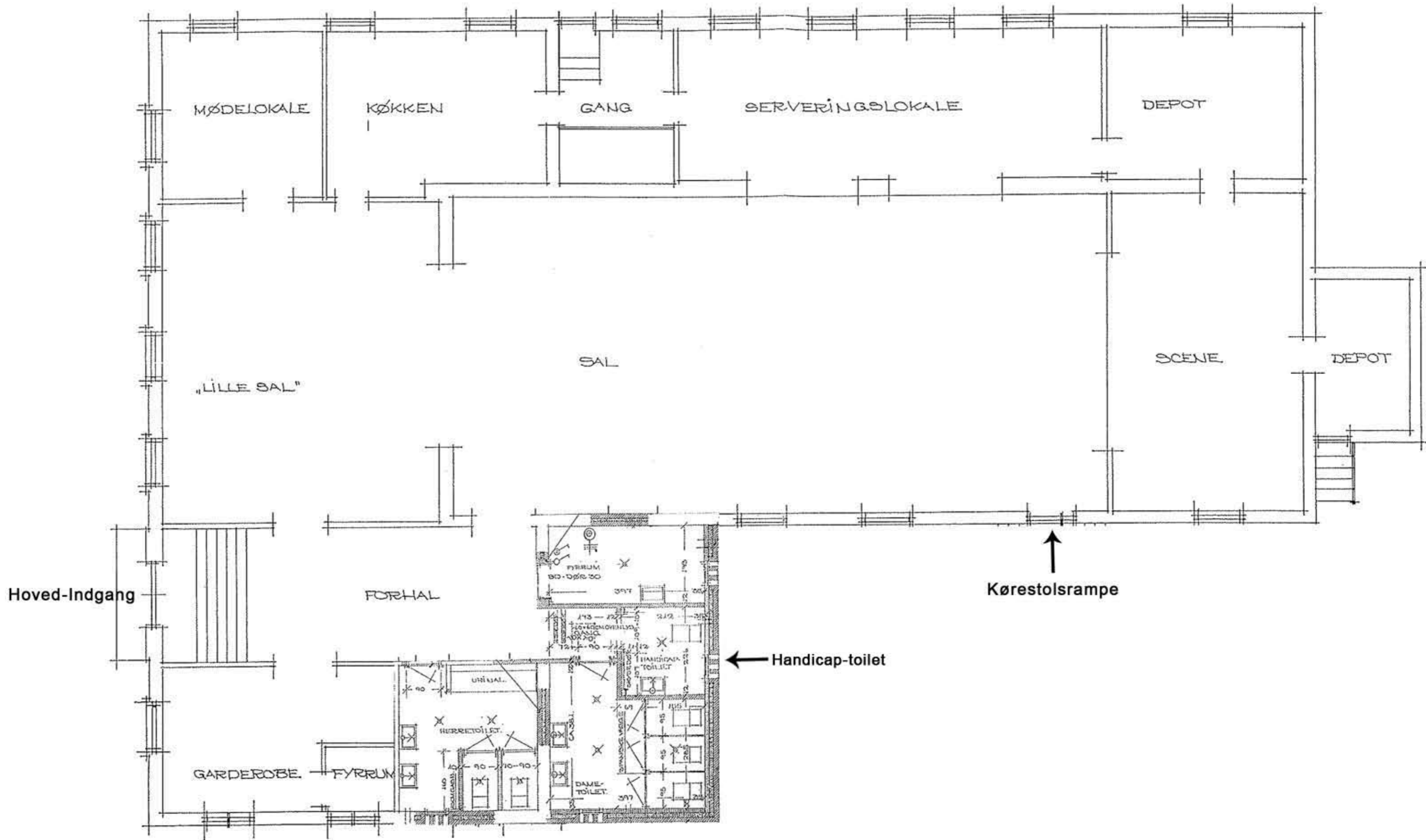
STUEPLAN ~ EKSIISTERENDE FORHOLD ~ MÅL 1:100.
